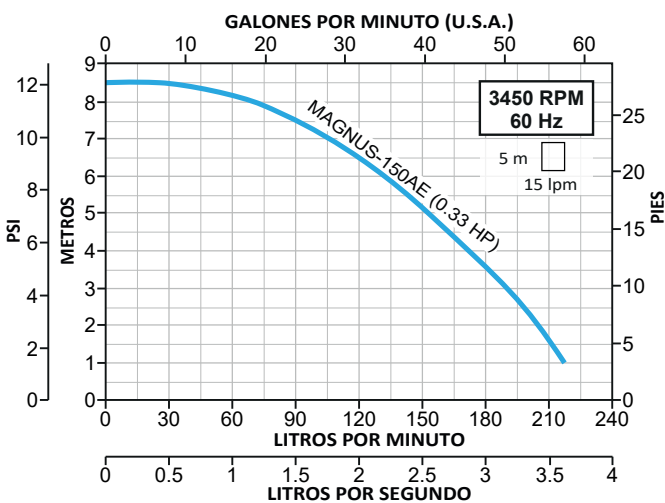
CURVA DE OPERACIÓN (MAGNUS-150AE)
